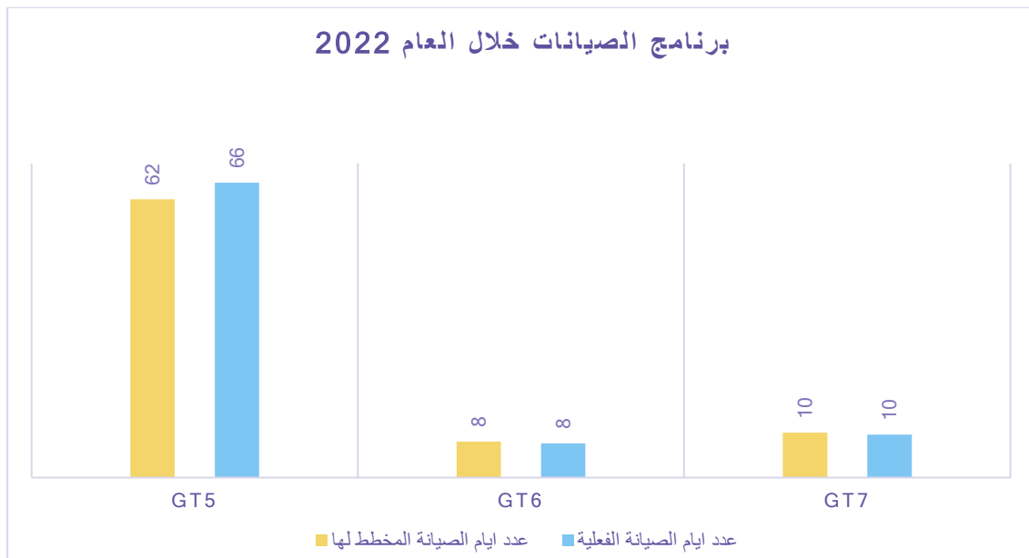
شكل (12) عدد أيام الصيانات للوحدات التوليدية
