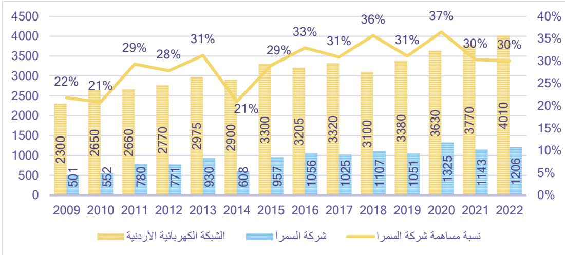
شكل (10) تطور الحمل الأقصى في الأردن و نسبة مشاركة السمرا
